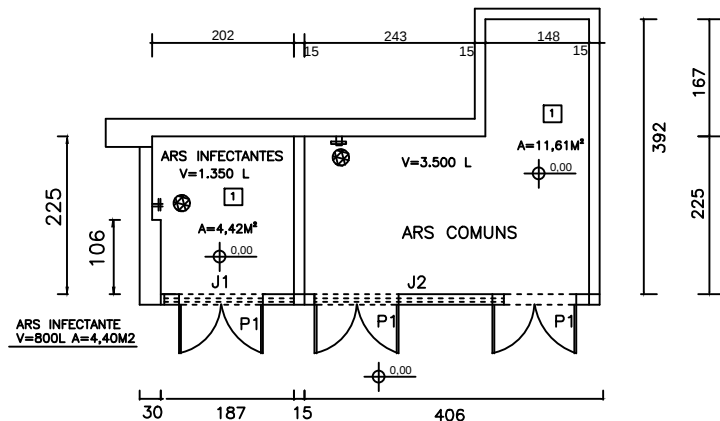
PLANTA BAIXA DOS ABRIGOS ESCALA.....1:50
