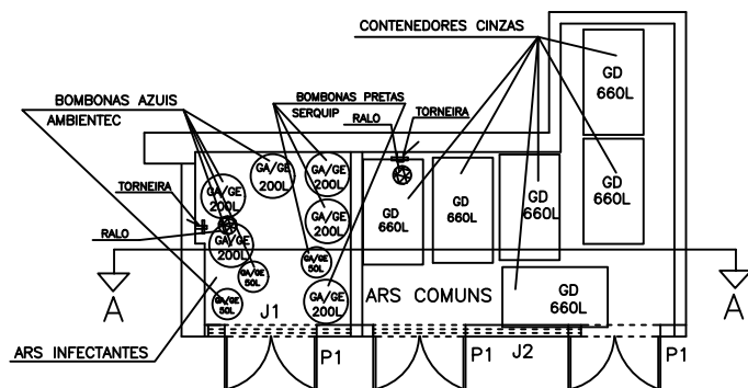
LAY OUT DOS ABRIGOS ESCALA.....1:50
